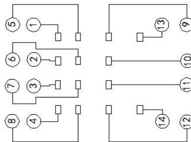
接线图
