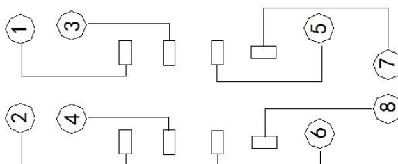
接线图
