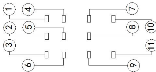
接线图
