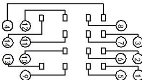
接线图
