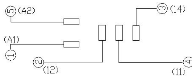
接线图
