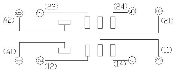
接线图
