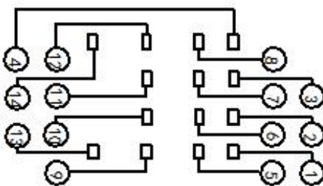
接线图
