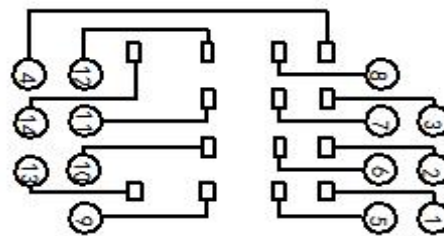
接线图
