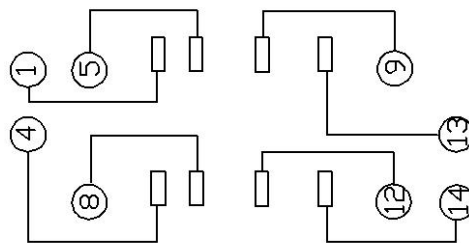
接线图
