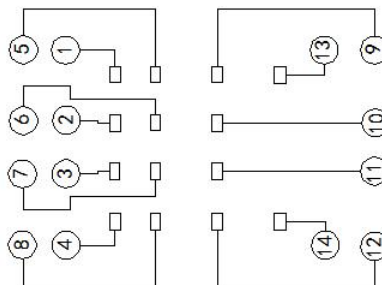
接线图
