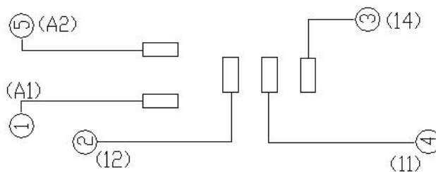
接线图
